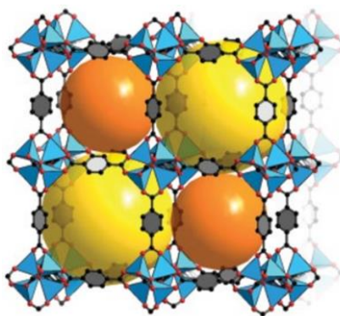
Slika 14. Struktura MOF-5: žute sfere = veće šupljine, narančaste sfere = manje šupljine, crno = C atomi, crveno = O atomi i plavi poliedri = Zn.
