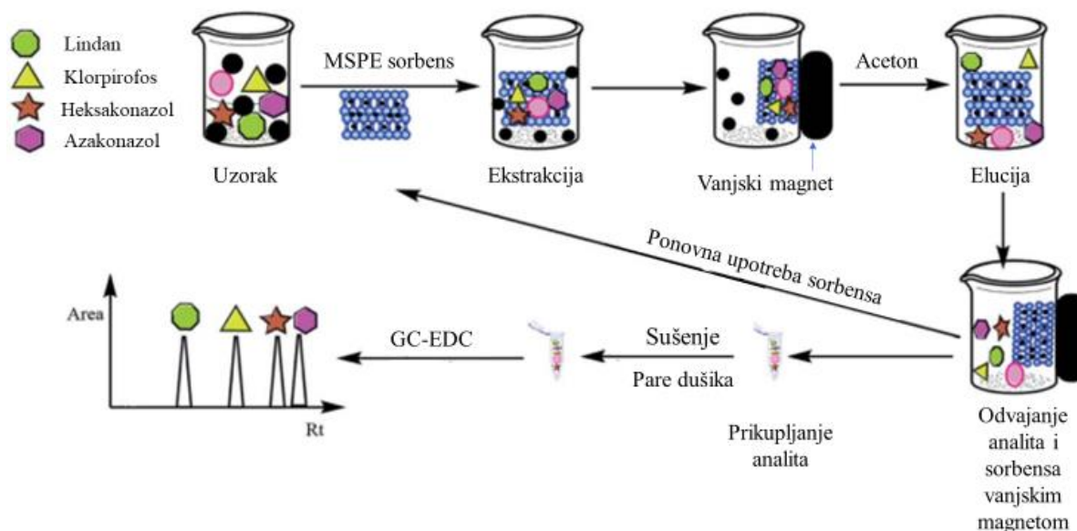
Slika 12. Postupak MSPE sa sorbensom \text{Fe}_3\text{O}_4/\text{SiO}_2\text{-G} za ekstrakciju organoklornih pesticida iz okolišnih voda. Preuzeto i prilagođeno iz ref. 55.
