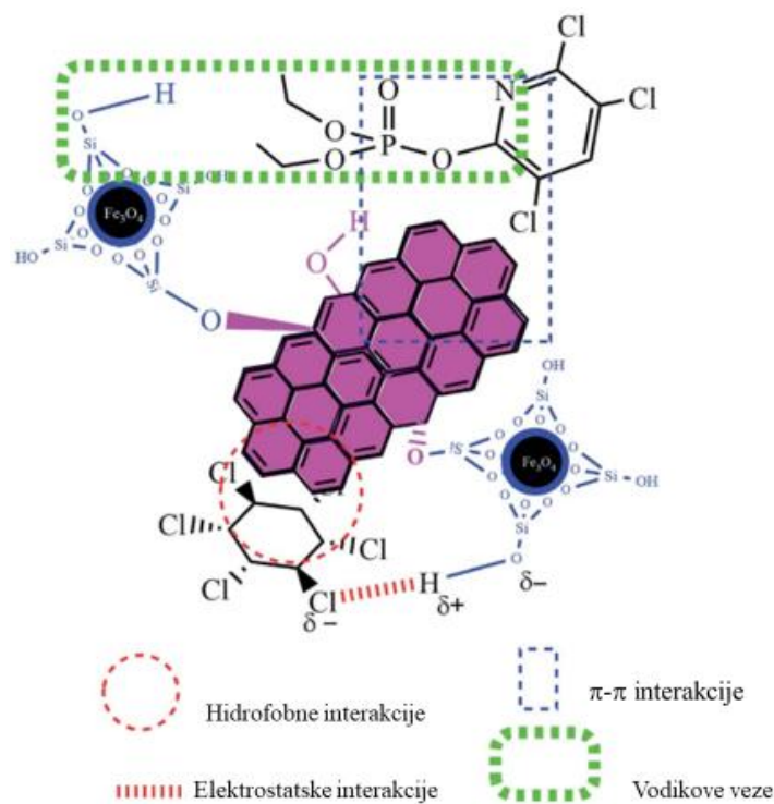
Slika 13. Interakcije pri adsorpciji organoklorinih pesticida na sorbensu pri MSPE. Preuzeto i prilagođeno iz ref. 55.
