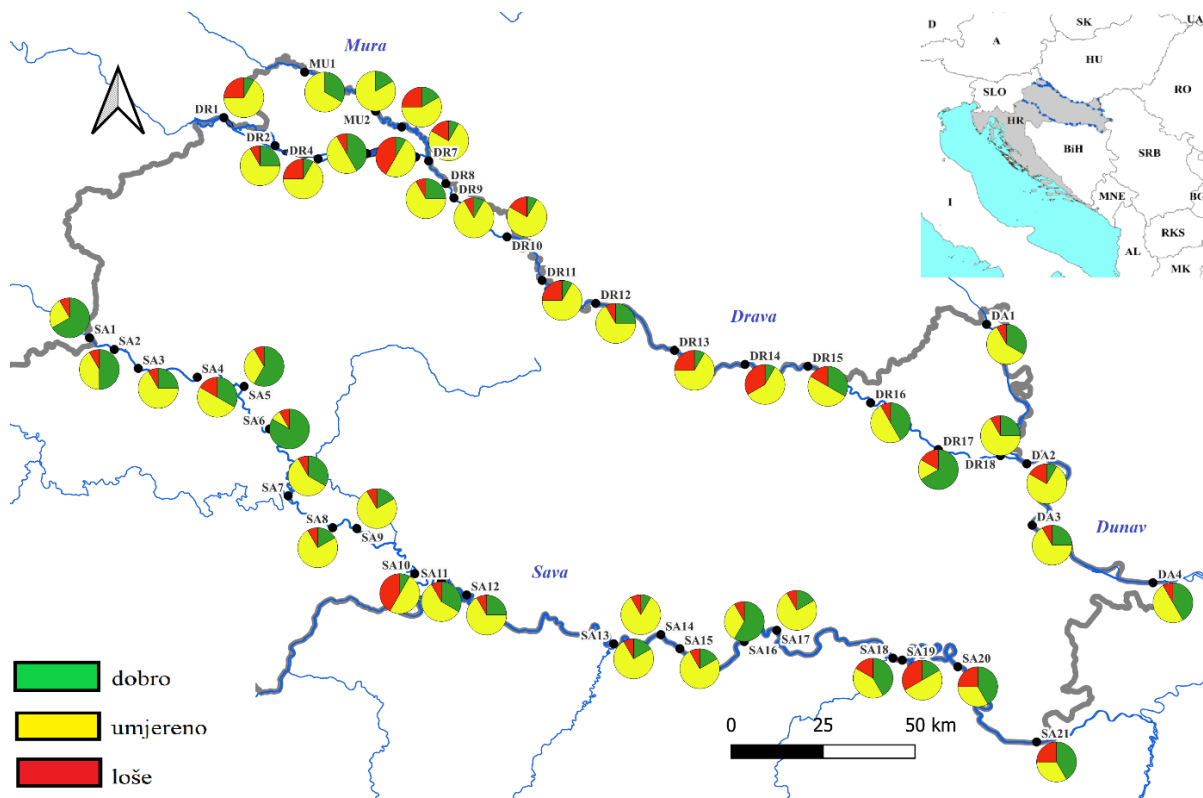
Slika 26. Udio stanja (dobro, umjereno, loše) na mjernim postajama na velikim rijekama (Sava, Mura, Dunav, Drava) u RH obzirom na: a) hranjive tvari (TN, TP). Lijeva polovica svakog kruga odnosi se na TP dok se desna odnosi na TN; b) koncentracije 11 metala (As, Cd, Co, Cr, Cu, Fe, Mn, Mo, Ni, Pb, Zn) u sedimentu. Šifre postaja nalaze se u Tablici 5.
