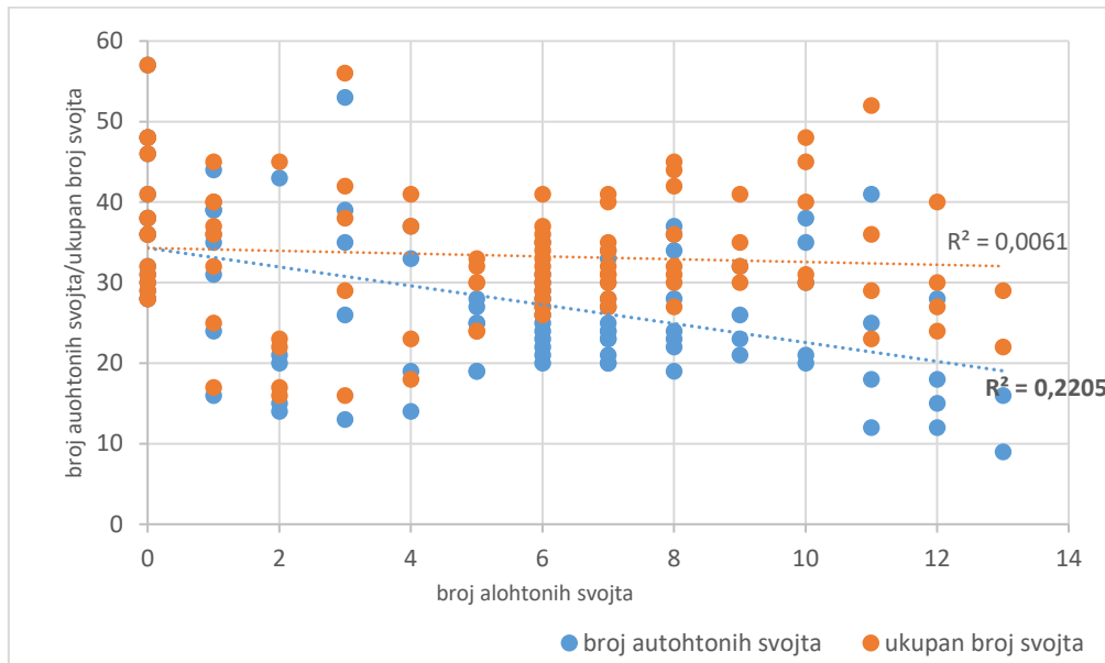
Slika 15. Odnosi između broja alohtonih vrsta makrozoobentosa i ukupnog broja svojti ili autohtonih svojti na svih 49 lokacija na velikim rijekama (Sava, Mura, Dunav, Drava) u RH s linijama koje predstavljaju linearnu regresiju (plava linija: broj autohtonih i broj alohtonih svojta; crvena linija: broj alohtonih svojta i ukupni broj svojta) i koeficijent determinacije R^2 (podebljano-značajne korelacije, p < 0,05 ).
