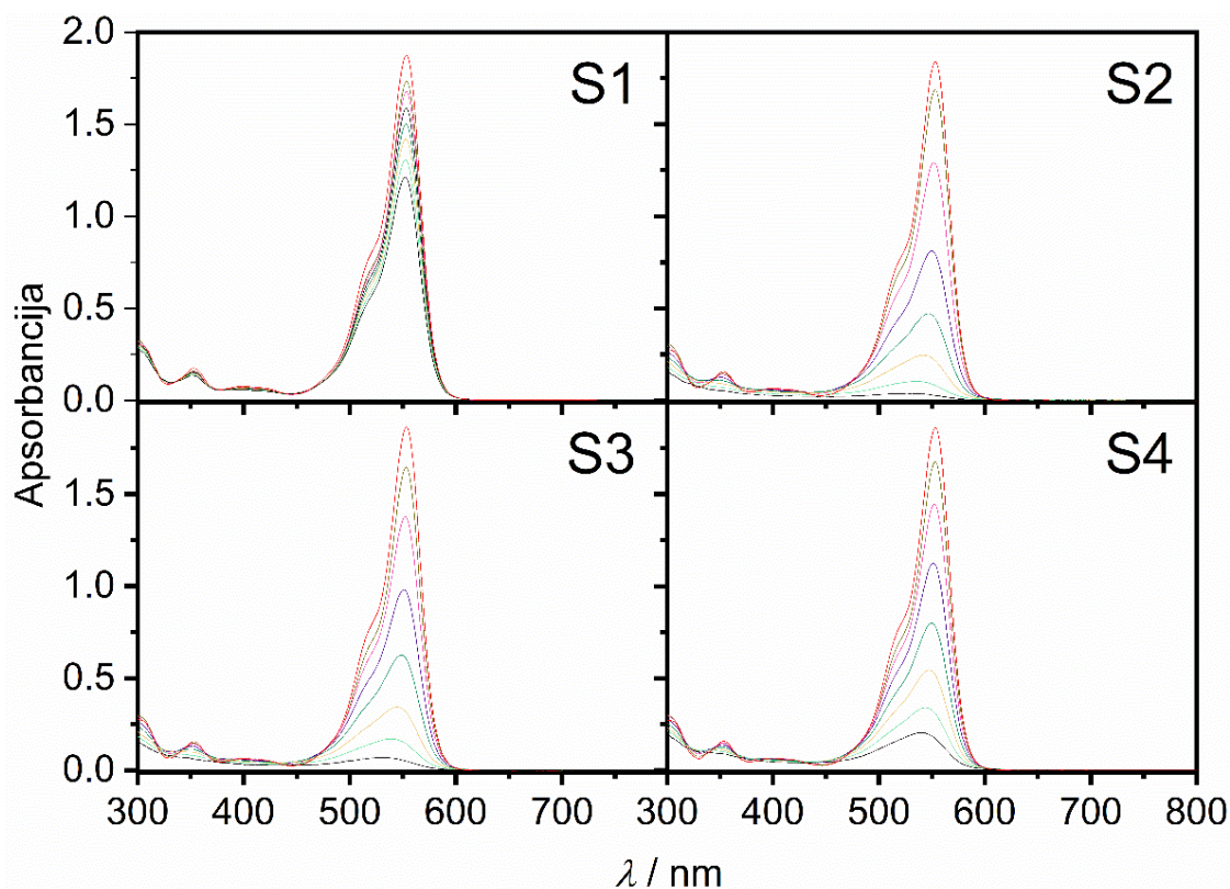
Slika 66. UV-Vis spektri otopina RhB tijekom fotokatalitičke evaluacije uzoraka S1-S4
