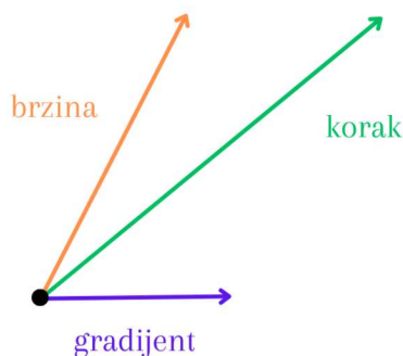
Slika 3.3: Metoda momentum
