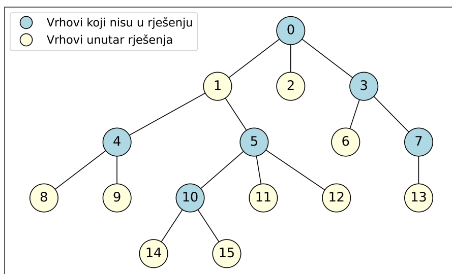
Slika 5.1: Primjer rješenja problema MWIS na stablima
