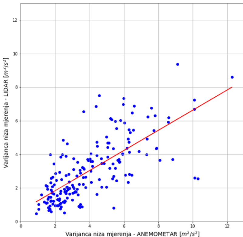
Slika 3.15. Ovisnost varijance niza mjerenja LIDAR-a o varijanci niza mjerenja anemometra za epizodu bure koja je trajala od 15:00 (21.3.2018.) do 19:00 (22.3.2018.) na području zračne luke Dubrovnik
