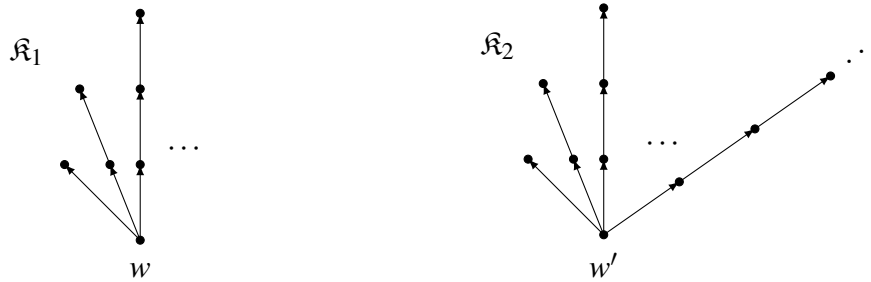
Slika 2.8: Svjetovi w i w' su modalno ekvivalentni, ali ne i bisimulirani
