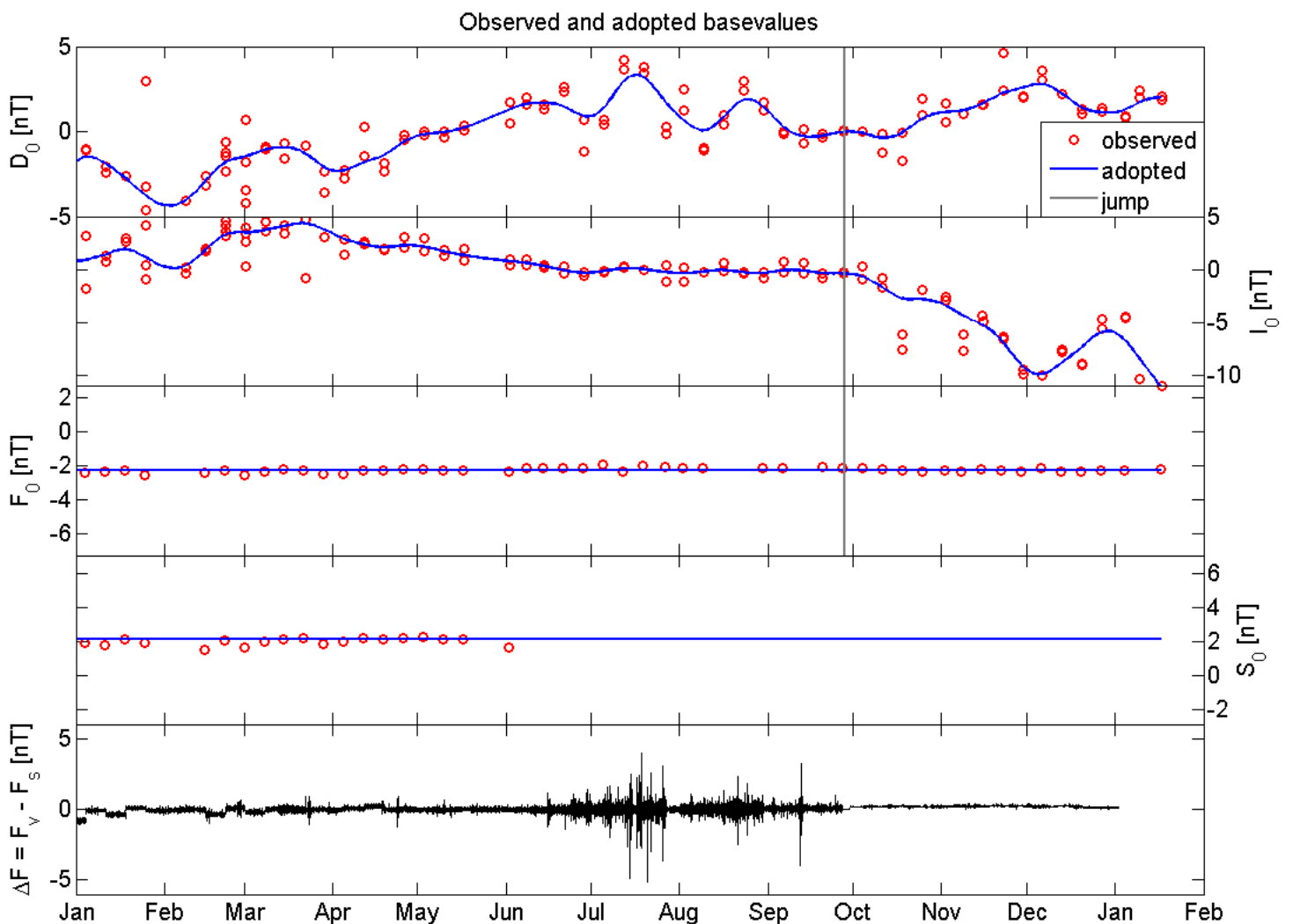
Slika 2.2 – Opažene ( engl. observed ) i prilagođene ( engl. adopted ) kalibracijske vrijednosti za DIDD variometar. Na slici su također prikazani rezultati motrenja s početka siječnja koji su korišteni u izračunu kalibracijskih krivulja za prosinac.
