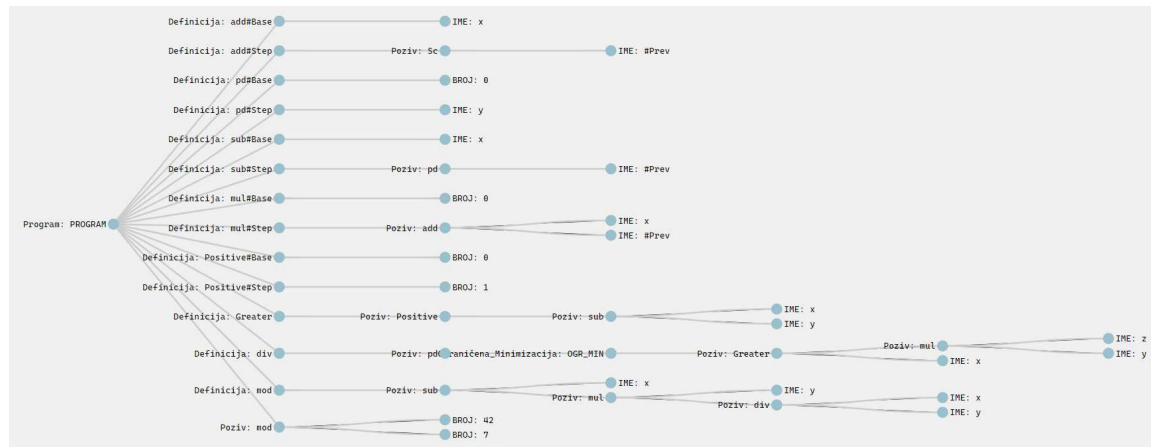
Slika 2.3: Stablo parsiranja
