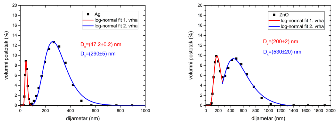
Slika 97. Grafički prikazi ovisnosti volumnog postotka po veličini koloidnih nanočestica srebra (a.) i cink oksida (b.) sa prilagodbom log-normalne raspodjele. Prikazani su medijan dijometri D_x obiju log-normalnih raspodjela.
