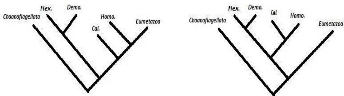
Slika 2. Parafiletsko (lijevo) i monofiletsko (desno) podrijetlo spužava, preuzeto i prilagođeno s https://u.osu.edu/eeob3320/2015/03/
