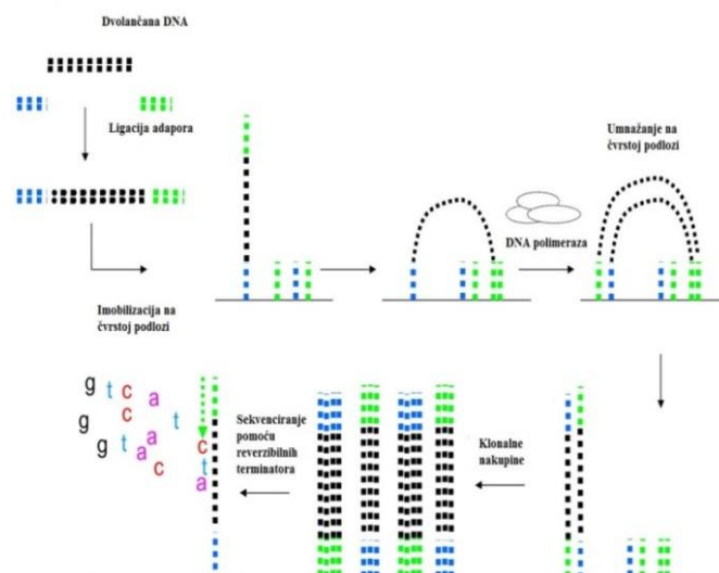
Slika 3. Shema sekvenciranja pomoću Illumine, preuzeto i prilagođeno s http://www.gsejournal.org/content/44/1/21/figure/F2?highres=y
