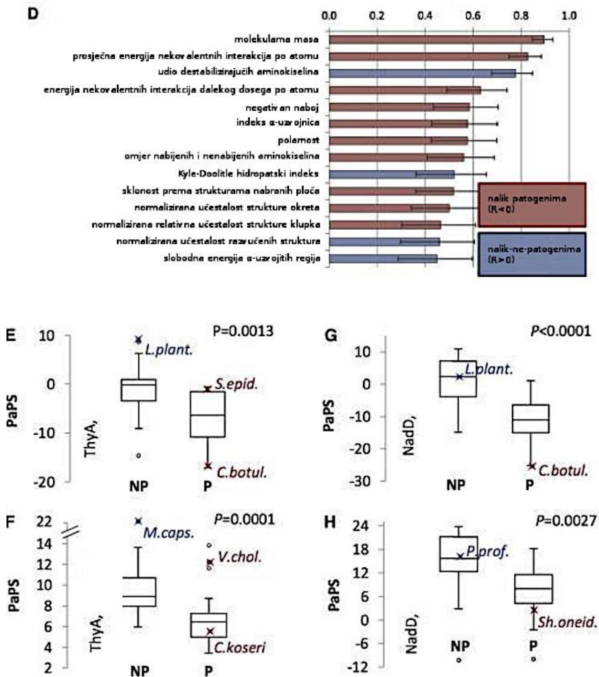
Slika 16. Dominantni trendovi u fizikalno-kemijskim svojstvima proteoma. (A i B) Kumulativni histogrami PaPS rezultata za patogene (crvena linija) i ne-patogene (plava linija). Proteomi patogena naginju prema nižim PaPS vrijednostima. Dmax je Kolmogorov-Smirnov (K-S) statistika, a p vrijednost je K-S test ("two-tailed"). (C) Standardizirani koeficijenti višestrukih linearnih regresija PaPS motiva naspram aminokiselinskim frekvencijama. * p < 0.001 (t test). (D) Najsnažnije korelacije između PaPS i seta aminokiselinskih fizikalno-kemijskih svojstava. Stupci pogrešaka u (C) i (D) su unutar intervala od 95% točnosti. (E–H) Distribucija PaPS rezultata unutar ThyA i NadD proteinskih familija, kontrastirana između patogena i ne-patogena; p vrijednosti dobivene two-tailed Mann-Whitney testom. Proteini odabrani za slijedeće eksperimente su označeni i skraćena imena vrsta su pokazana. Vrijednost koja odstupa u setu patogena u (F) zahtijeva dodatna razjašnjenja.
