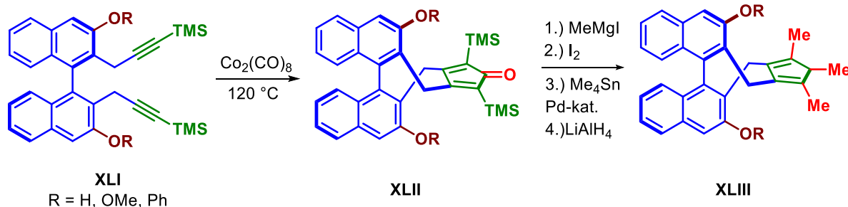
Slika 13. Sinteza pentasupstituiranih kiralnih ciklopentadiena s binaftalenskom okosnicom.
