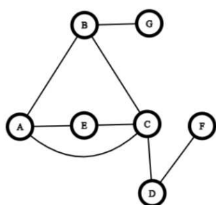
Slika 2.5: Graf G
