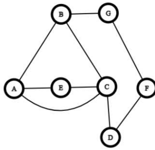
Slika 2.6: Graf G + \{F, G\}
