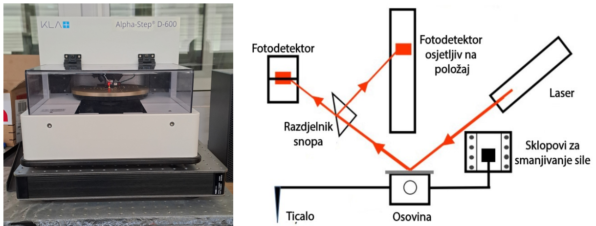
Slika 5.12: Lijevo: KLA Alpha Step D-600 kontaktni profilometar koji smo koristili. Desno: Shema kontaktnog profilometra. Preuzeto s izvora [48] i prilagođeno.
