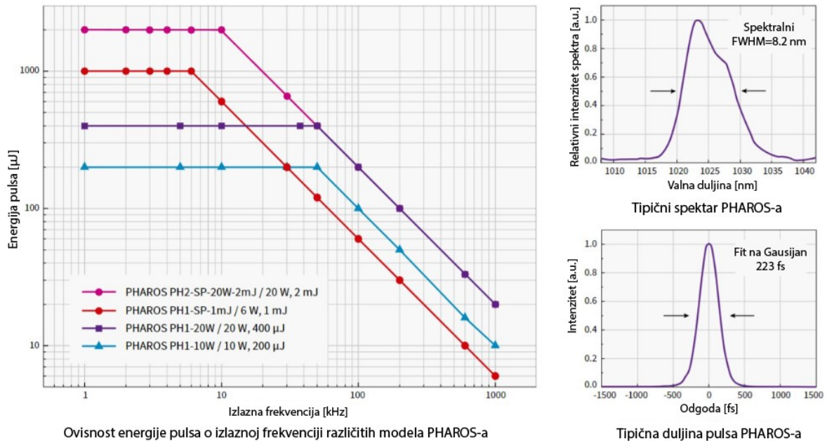
Slika 5.7: Lijevo: Ovisnost energije pulsa o izlaznoj frekvenciji za različite modele PHAROS lasera. Desno gore: Prikaz tipičnog spektra PHAROS lasera. Desno dolje: Prikaz tipične duljine pulsa PHAROS lasera. Preuzeto s izvora [39] i prilagođeno.
