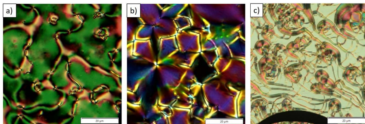
Slika 28. Teksture parnih dimera dobivenih hlađenjem uzorka: a) schlieren tekstura N faze spoja BB-8-BB pri 116 °C, b) focal-conic tekstura N^* faze spoja (S)-BB-6-BB pri 125 °C; c) tekstura uljnih pruga N^* faze spoja (S)-BB-8-BB pri 112 °C.
