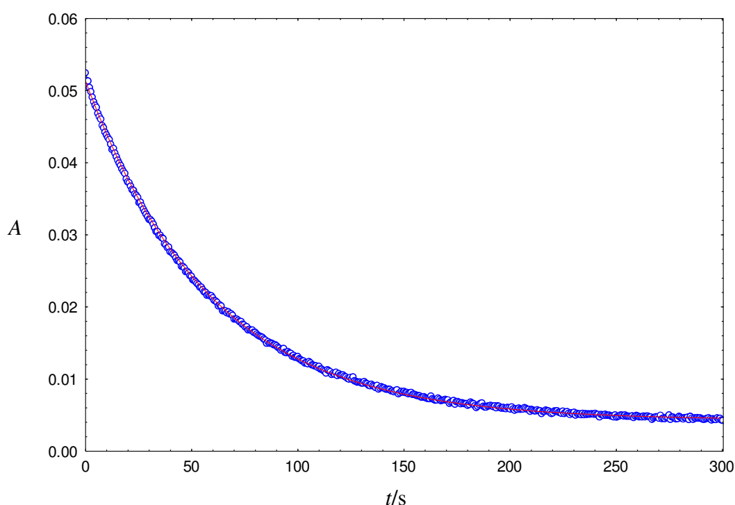
Slika 3.2. Promjena apsorbancije heksacijanoferat (III) iona na 420 nm (plavi kružići) u vremenu, u reakciji askorbata i heksacijanoferata(III) u smjesi otapala acetonitril : \text{H}_2\text{O} = 1 : 1 v/v, na 298 K. c(\text{NaHAsc}) = 0,0005 \text{ mol dm}^{-3} , c(\text{K}_3[\text{Fe}(\text{CN})_6]) = 0,00005 \text{ mol dm}^{-3} , c(\text{Na}_2\text{EDTA}) = 0,0005 \text{ mol dm}^{-3} ; I_c = 0,0023 .
