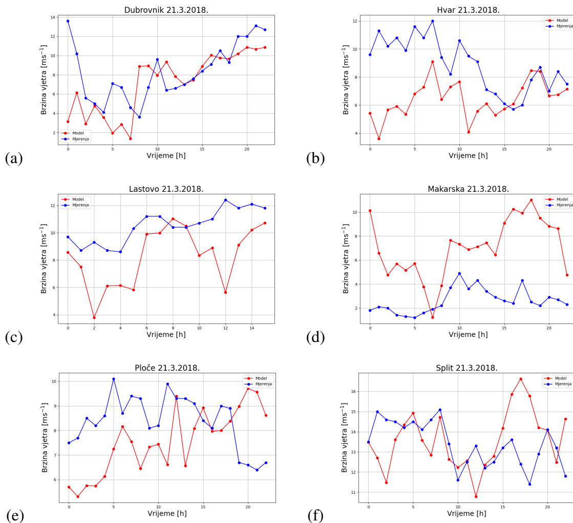
Slika 3.29. Usporedba izmjerenih (plavo) i modelski (crveno) dobivenih vrijednosti brzine vjetra na 10 m visine na svim mjernim postajama osim Splita za slučaj 21.3.2018.
