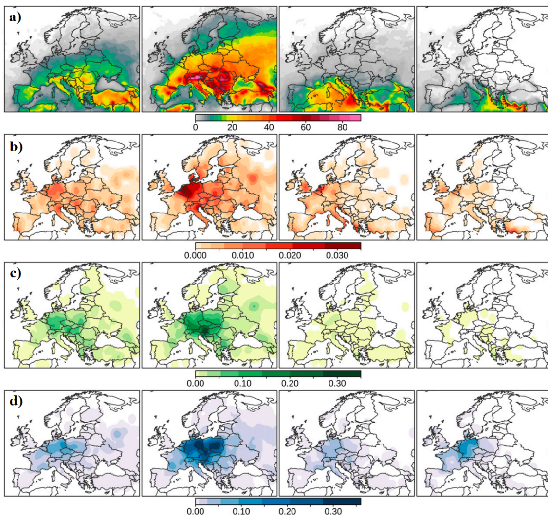
Slika 1.4. Prosječni broj sati s; (a) munjama, (b) tornadima, (c) velikom tučom, (d) jakim udarima vjeta na mreži točaka s udaljenošću od 0.25^\circ nakon prostornog filtriranja za Europu u razdoblju od 2006. do 2018. godine po sezonama (proljeće, ljeto, jesen, zima; slijeva nadesno) (Taszarek i sur., 2020.)
