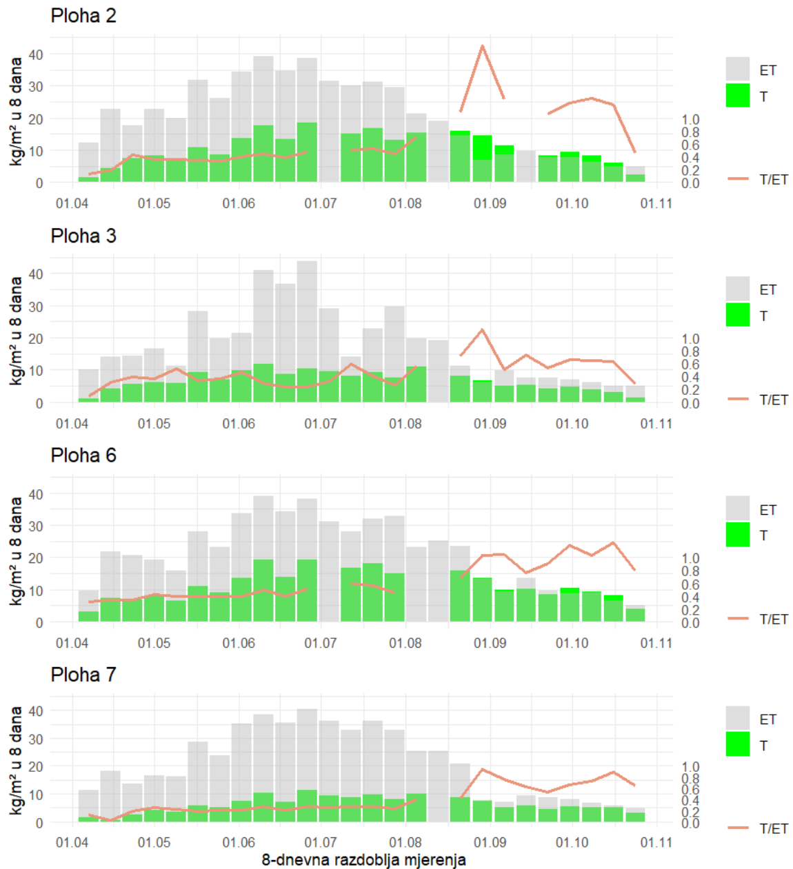
Slika 30. Usporedni prikaz dinamike MODIS evapotranspiracije (ET) (8-dnevni zbroj) i protoka ksilemskog soka (T) izmjenjenog na terenu (na razini sastojine, 8-dnevni zbroj) za travanj-listopad 2019. Na dane kad terenski mjereni podaci za transpiraciju nisu bili cjeloviti (npr. nedostajali su potpuni podaci za cijeli dan), cijeli 8-dnevni period nije imao procjenu transpiracije. Vrijednosti omjera T/ET prikazane su na sekundarnoj y-osi.
