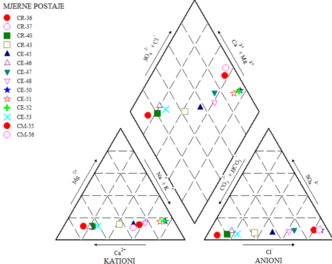
Slika 11. Piperov trilinearni dijagram s hidrokiemijskim facijesima donjeg toka i estuarija rijeke Cetine.
