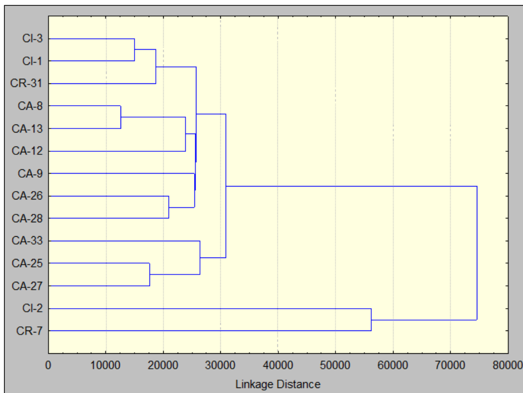
Slika 29. Klastera analiza ispitivanih mjesta uzorkovanja, ali prema sadržaju elemenata u površinskom sedimentu frakcije < 63 µm gornjeg i srednjeg toka rijeke Cetine.
