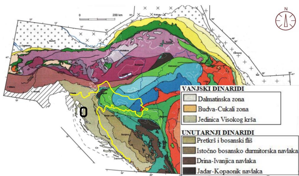
Slika 1. Tektonske jedinice Vanjskih i Unutarnjih Dinarida. Istraživano područje Vinodolske doline označeno je crnom oznakom na karti (modificirano prema SCHMID i sur., 2008)
