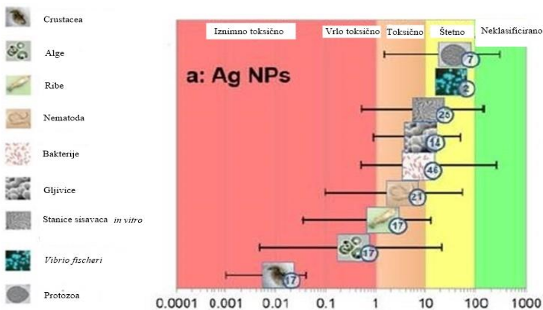
Slika 24. Piktogram medijana EC 50 vrijednosti ± minimalne i maksimalne vrijednosti (iz većeg broja istraživanja) za testne vrste s pripadajućom legendom. Na x-osi su koncentracije nanosrebra u mg Ag/L. Različite boje unutar piktograma predstavljaju kategorizaciju toksičnosti prema EU-Direktivi 93/67/EEC (preuzeto i prilagođeno iz Bondarenko i sur., 2013.).
