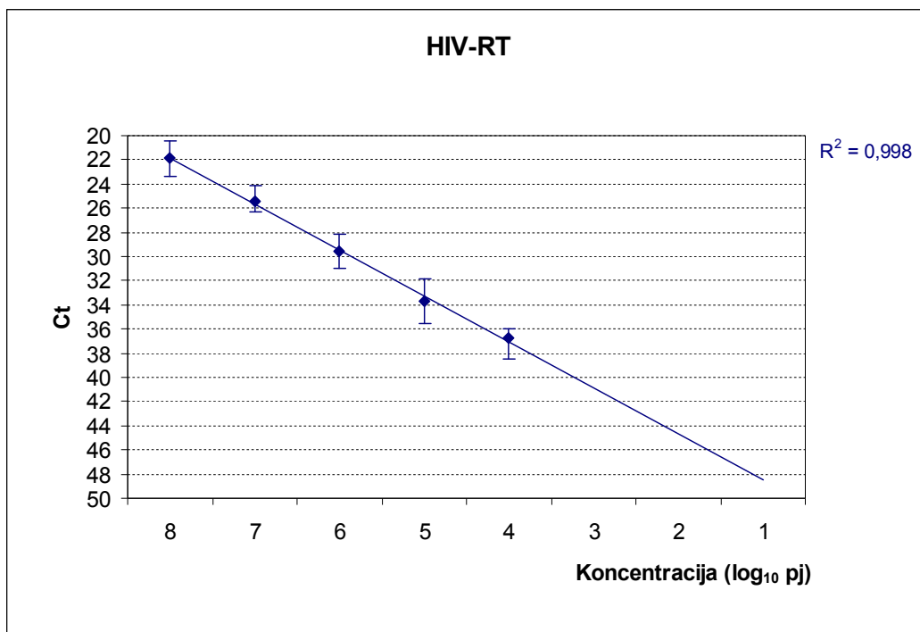
Slika 18. Srednja vrijednost Ct za HIV-RT u tri PERT-testa ( \bar{X}_{n_r} , Tablica 9.). Stupci pogreške predstavljaju raspon Ct iz svih testiranja pojedine koncentracije RT. Povučen je regresijski pravac i određen koeficijent determinacije.
