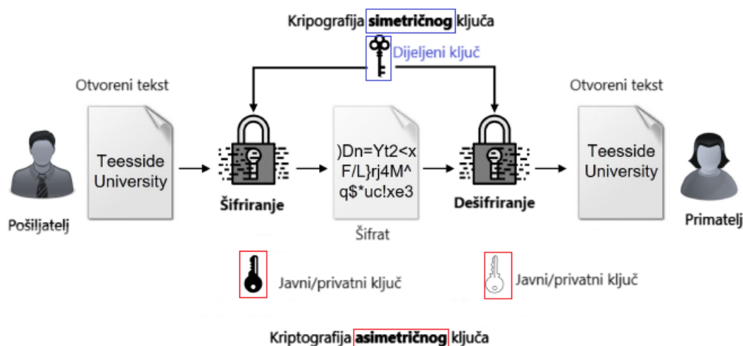
Slika 2.3: Glavni tipovi kriptografije [24]
