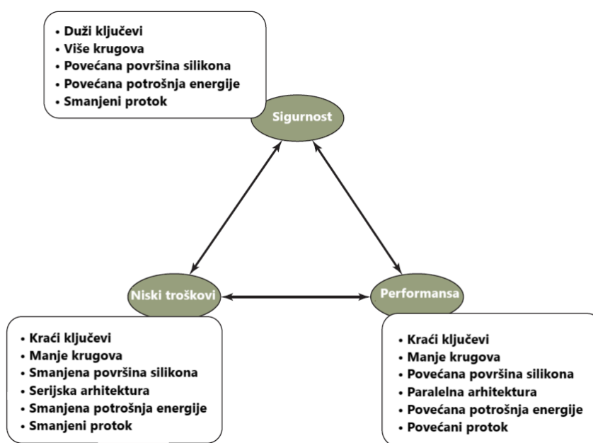
Slika 2.9: Kompromisi u lakoj kriptografiji
