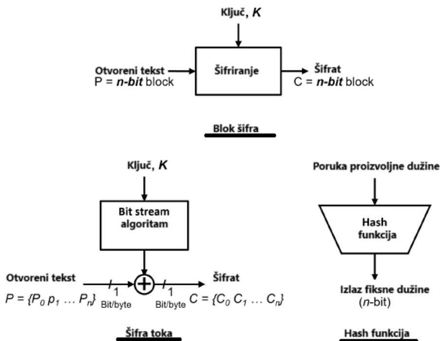
Slika 2.4: Blok šifra, šifra toka i hash funkcija
