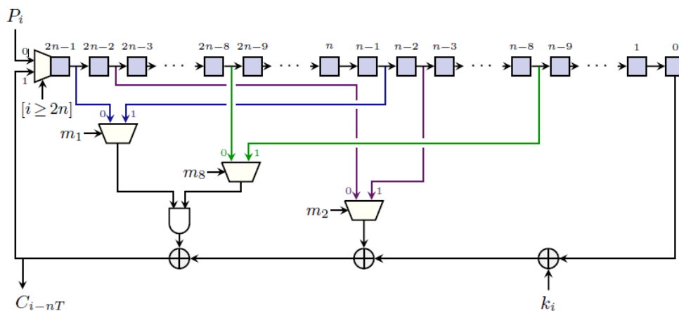
Slika 3.11: Serijalizacija Simon funkcije runde, jedan bit u isto vrijeme [4]
