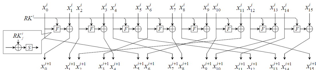
Slika 3.19: Rundna funkcija Twine algoritma [23]
