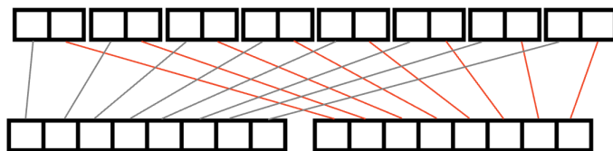
Slika 3.18: Podjela otvorenog teksta prije rundne funkcije
