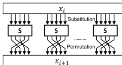
Slika 3.1: SPN [24]
