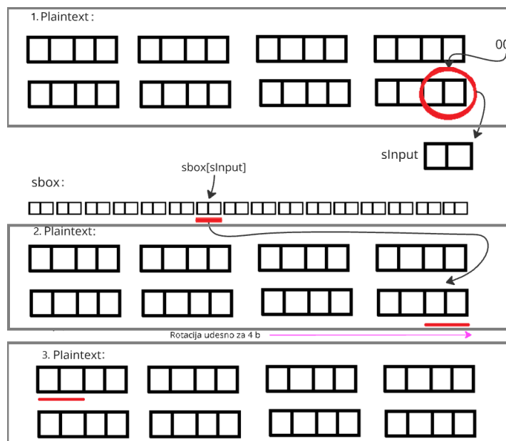
Slika 3.5: SBoxLayer
