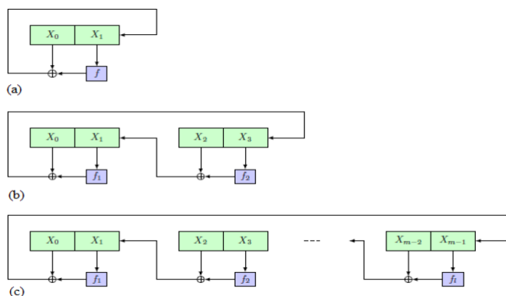
Slika 3.9: Feistelova struktura s različitim duljinama [10]
