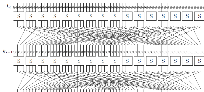
Slika 3.4: SP mreža za Present [5]
