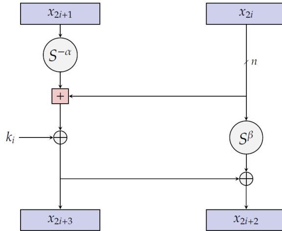
Slika 3.15: Struktura Speck algoritma [2]
