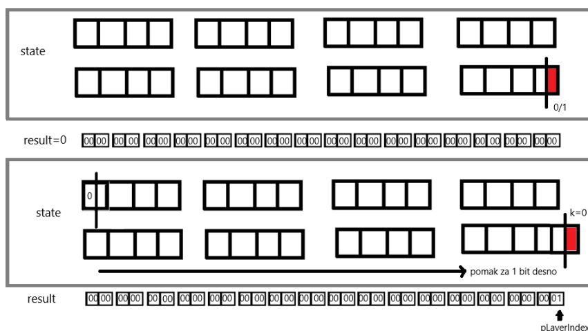
Slika 3.6: PermutationLayer
