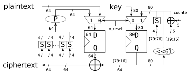
Slika 3.7: Present [5]
