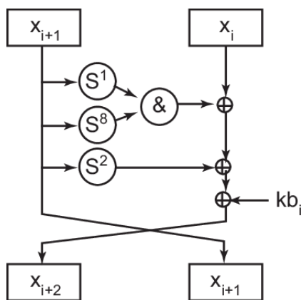
Slika 3.14: Feistelova funkcija [7]
