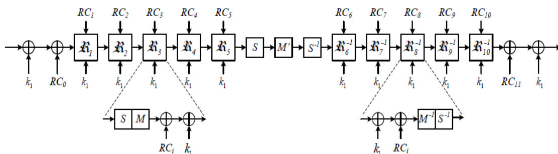
Slika 3.26: PRINCE core [6]
