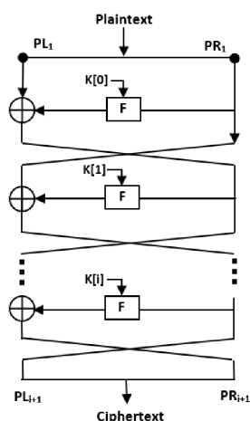
Slika 3.8: Feistel struktura [14]
