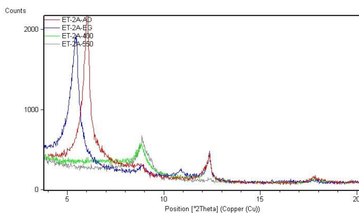
Slika 36. Prikaz usporednih rendgenograma orijentiranih preparata za uzorak ET-2A sušenih na zraku (ET-2A-AD), bubrenih etilen-glikolom (ET-2A-EG), žarenih na 400° C (ET-2A-400) i žarenih na 550°C (ET-2A-550).
