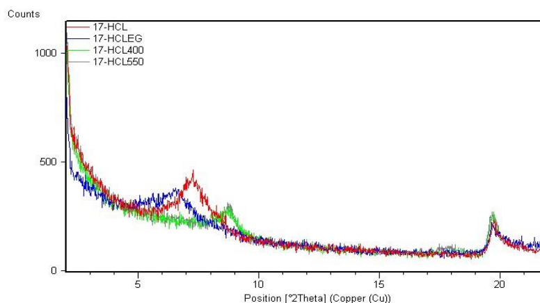
Slika 45. Prikaz usporednih rendgenograma orijentiranih preparata sušenih na zraku nakon tretiranja s HCl (17-HCL), bubrenih etilen-glikolom (17-HCLEG) žarenih na 400° C (17-HCL400) i žarenih na 550° C (17-HCL550) za uzorak 17.
