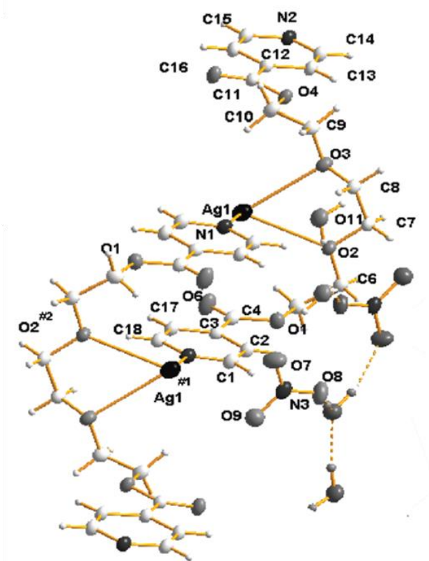
Slika 23. Struktura kompleksa \{[Ag(LI)NO_3]\}_n \cdot 2H_2O .
