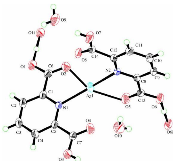
Slika 15. Koordinacijska sfera srebrova(I) iona u [Ag(C_7H_4NO_4)(C_7H_5NO_4)] \cdot 2H_2O .
