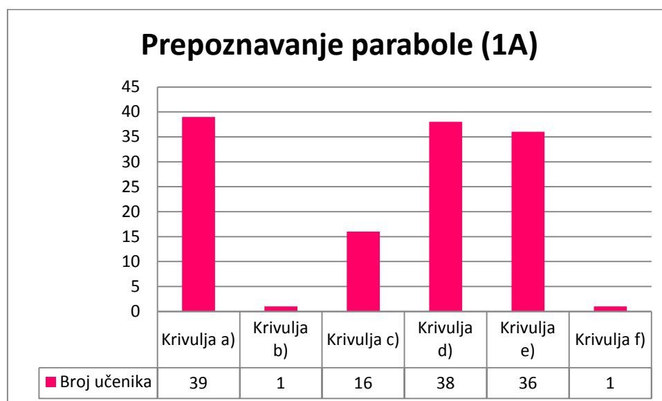
Slika 4.2. Dijagram frekvencija – Prepoznavanje parabole (1A)
