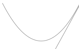
Slika 3.3.4. Pravac i parabola iz zadatka 5. – posttest
