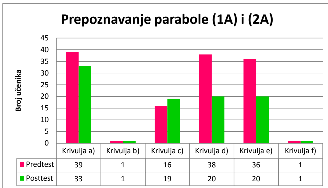
Slika 4.13. Dijagram usporedbe rezultata pretesta i posttesta
