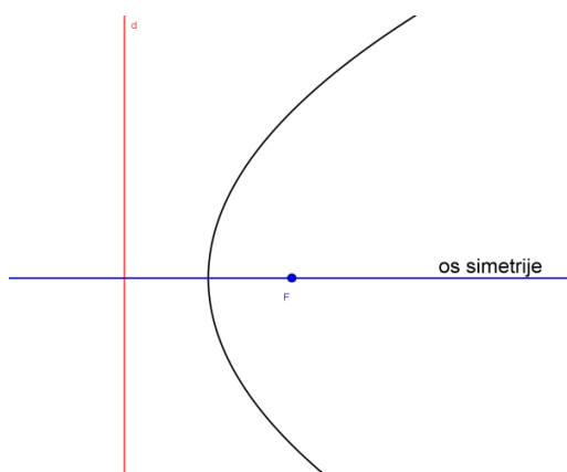
Slika 5.4.2. Pravac simetrije kod parabole
