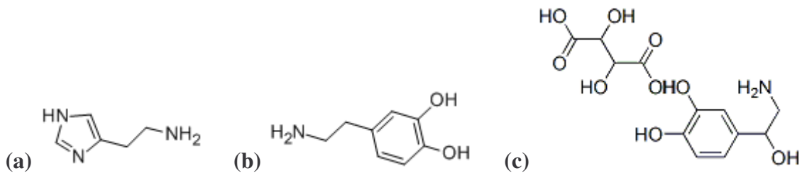
Slika 5. Strukture nekih od glavnih peptidnih sastavnica iz pčelinjega otrova: melitin (a), apamin (b), peptid koji degranulira mastocite (c), sekapin (d) i terciapin (e) (slike preuzete sa internetske stranice http://www.chemicalbook.com ).
