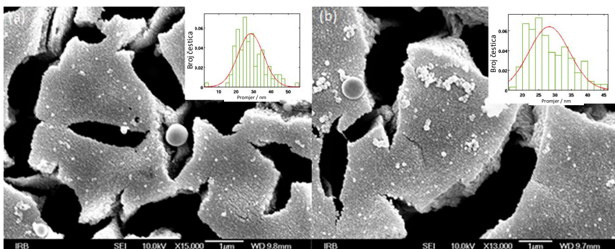
Slika 65 SEM slike uzoraka poroznog Si nakon ablacije sa zlatom: a) uzorak #2 (povećanje 15 000 \times ) i c) uzorak #3 (povećanje 13 000 \times ) s odgovarajućim raspodjelama veličine čestica (umetci).
