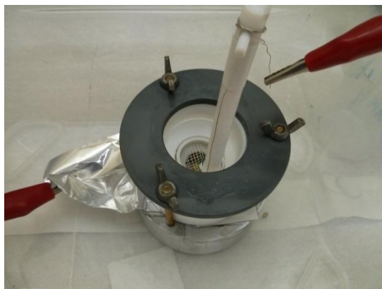
Slika 61 Čelija za elektrokemijsko jetkanje silicija (napravljena u Laboratoriju za molekulska fiziku, IRB) za vrijeme jetkanja.
