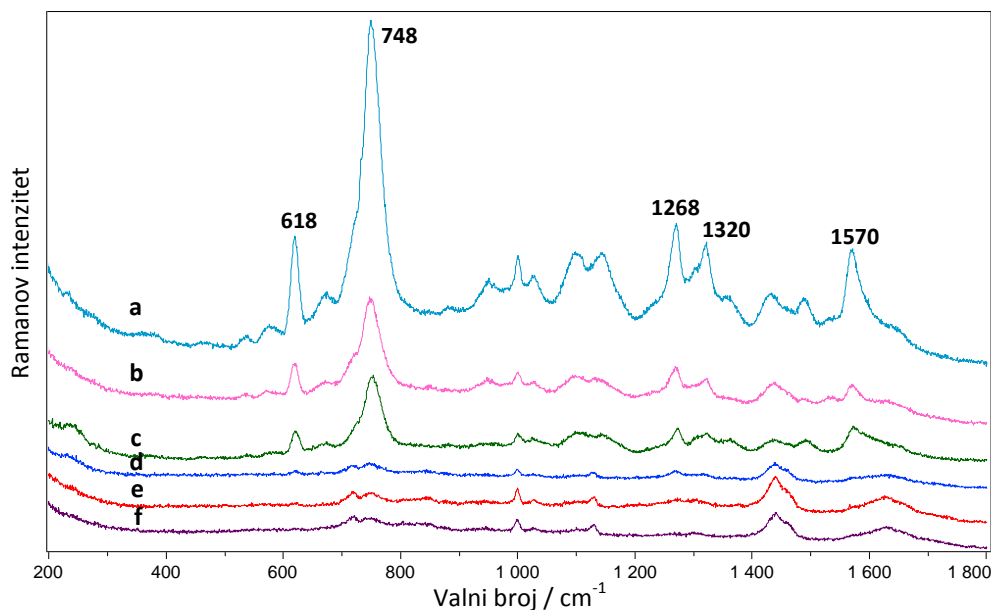
Slika 90 SERS spektri različitih koncentracija histamina u AGC koloidnoj suspenziji: a) 10 -2 M, b) 10 -3 , c) 10 -4 , d) 10 -5 , e) 5 × 10 -6 i f) voda (514,5 nm; 60 s).
