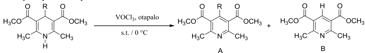
Tablica 50. Dealkilacija 2,6-dimetil-3,5-di(metoksikarbonil)-4-alkil-1,4-DHP s \text{VOCl}_3 pri sobnoj temperaturi i pri 0^\circ\text{C} .
