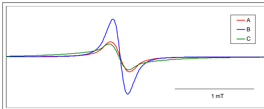
Slika 58: Eksperimentalni EPR spektar DDQ •- radikal aniona dobiven prilikom aromatizacije s DDQ A – spoj 1 + DDQ, B – spoj 21 + DDQ, C – spoj 2a + DDQ
