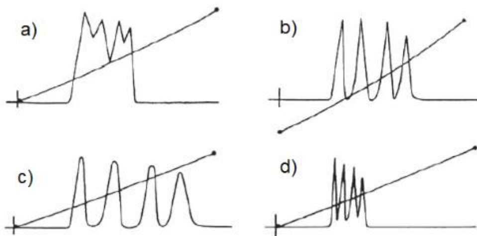
Slika 2. Primjeri kromatograma dobiveni b) smanjenjem udjela organske faze, c) smanjenjem nagiba gradijenta, d) povećanjem protoka. Kromatogram pod a) prikaz je razdvajanja prema početnim uvjetima. Preuzeto od Kromidas, 2006.
