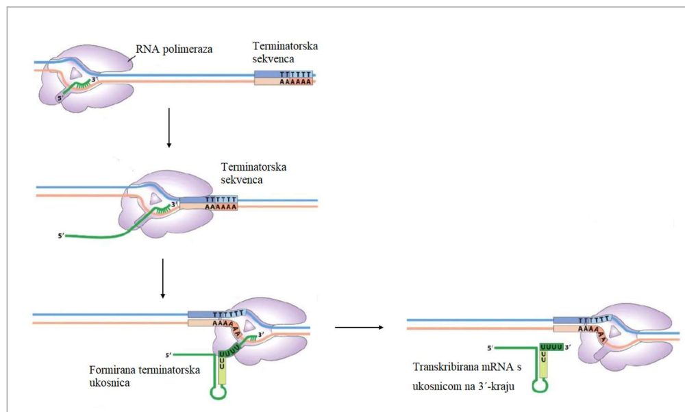
Slika 4. Shematski prikaz terminacije transkripcije ρ-neovisnim mehanizmom (Preuzeto i prilagođeno prema Ref. (3))
