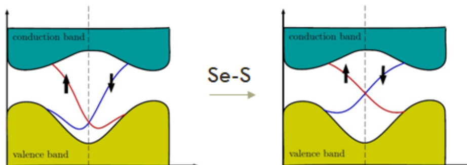
Slika 4.10: Shematski prikaz pomicanja Diracove točke zamjenjivanjem selenija sumporom. Diracova se točka energetske pomiče od stanja valentne vrpce pa su efekti topološkog izolatora izraženiji.
