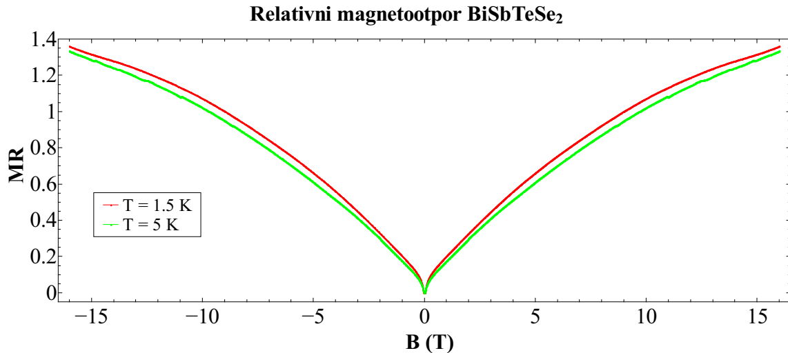
Slika 6.9: Relativni magnetootpor za BiSbTeSe_2 . Na nižoj temperaturi je izmjeren veći porast u magnetootporu mjenog uzorka. Kao kod BiSbTe_2S se iz logaritamske ovisnosti prepoznaje weak anti-localization efekt.
