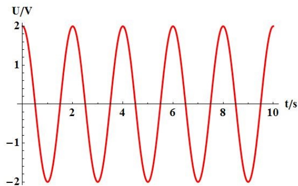
Slika 10.7: Ovisnost napona na kondenzatoru U o vremenu t .
