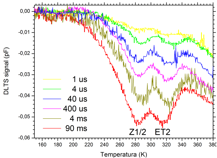
Slika 5.21: DLTS mjerenja na BN13 uzorku pri označenim širinama pulsa t_P . Iznos reverznog napona pri mjerenjima je V_R = -10 \text{ V} , naponskog pulsa V_P = -0.1 \text{ V} te perioda ponavljanja pulsa 1 \text{ s} .
