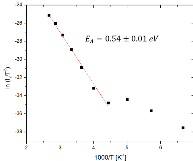
Slika 13: Richardsonov graf i određivanje aktivacijske energije za transport naboja u Si diodi
