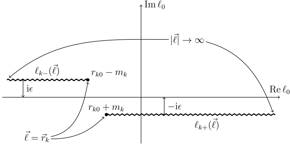
Slika 2.2: Singularna struktura jednog Feynmanovog propagatora. Valovite linije predstavljaju sve moguće položaje singulariteta u kompleksnoj \ell_0 ravni. Točan položaj singulariteta ovisi o trovektoru \vec{\ell} . Na ovoj je slici uzeto r_{k0} < -m_k , te \epsilon \approx 0 .
