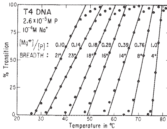
Slika 1.9: Krivulje prijelaza T4 DNA ( 2.6 \cdot 10^{-5} M DNA fosfata, 10^{-4} M \text{Na}^+ ) za različiti omjer dodatnih \text{Mg}^{2+} naspram fosfata DNA ( \text{Mg}^{2+}/\text{P} ). Omjer je naznačen uz uzorke a odmah ispod je naznačen nagib prijelaza očitana na temperaturi prijelaza.
