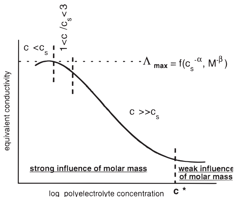
Slika 1.22: Generalna ovisnost ekvivalentne vodljivosti o koncentraciji polielektrolita za polimere udaljenosti naboja manje od Bjerrumove duljine ( b < l_b ). Eksperimentalni uvjeti: 5 \cdot 10^{-7} M < c < 10^{-2} M ; 10^{-6} M < c_s < 10^{-4} M . Preuzeto iz [13].
