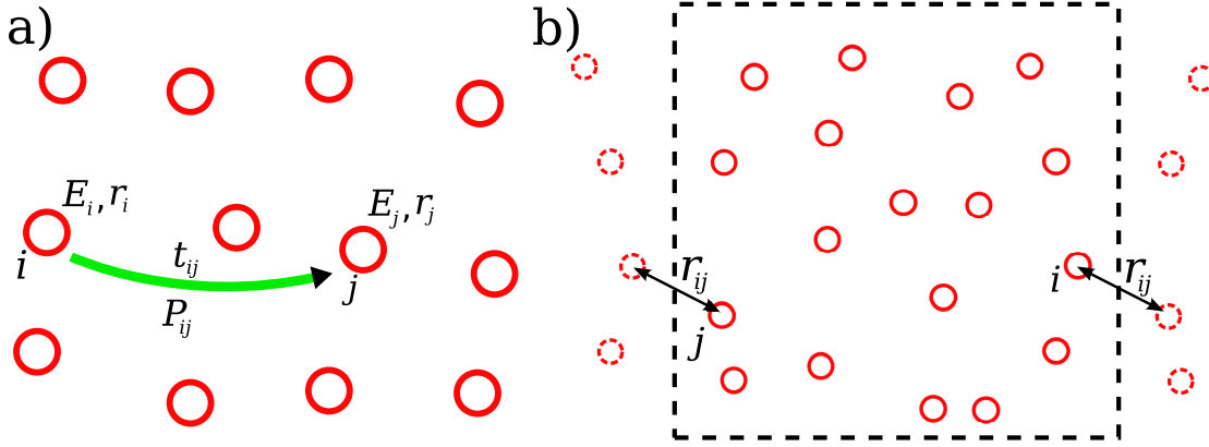
Slika 2.1: (a): Skica osnovnog modela. (b): Periodični rubni uvjeti (u 2D). Označena je minimalna udaljenost između čvorovišta i i j .
