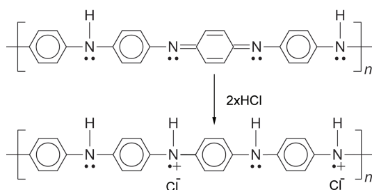
Slika 2.4: Prikaz neredoks dopiranja emeraldinske baze polianilina s \text{HCl} . Dopiranjem dolazi do strukturnih promjena u kralježnici polimera te stvaranja emeraldinske soli. Protu-ion \text{Cl}^- je ionski vezan na aminski kation dušika i osigurava nabojnu neutralnost.[20]
