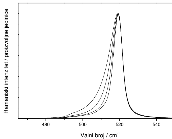
Slika 3.13. Ramanov intenzitet optičkog fonona izračunat po modelu kvantnog zatočenja uz istu srednju vrijednost čestica, ali s povećavanjem širine distribucije.
