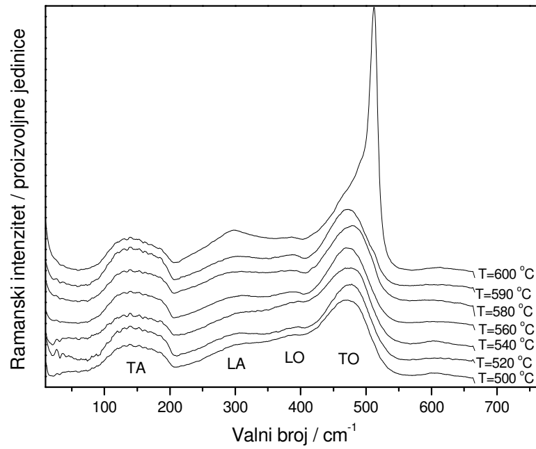
Slika 4.2. HH Ramanovi spektri uzoraka amornog silicija deponiranih na temperaturama od 500 do 600 °C
