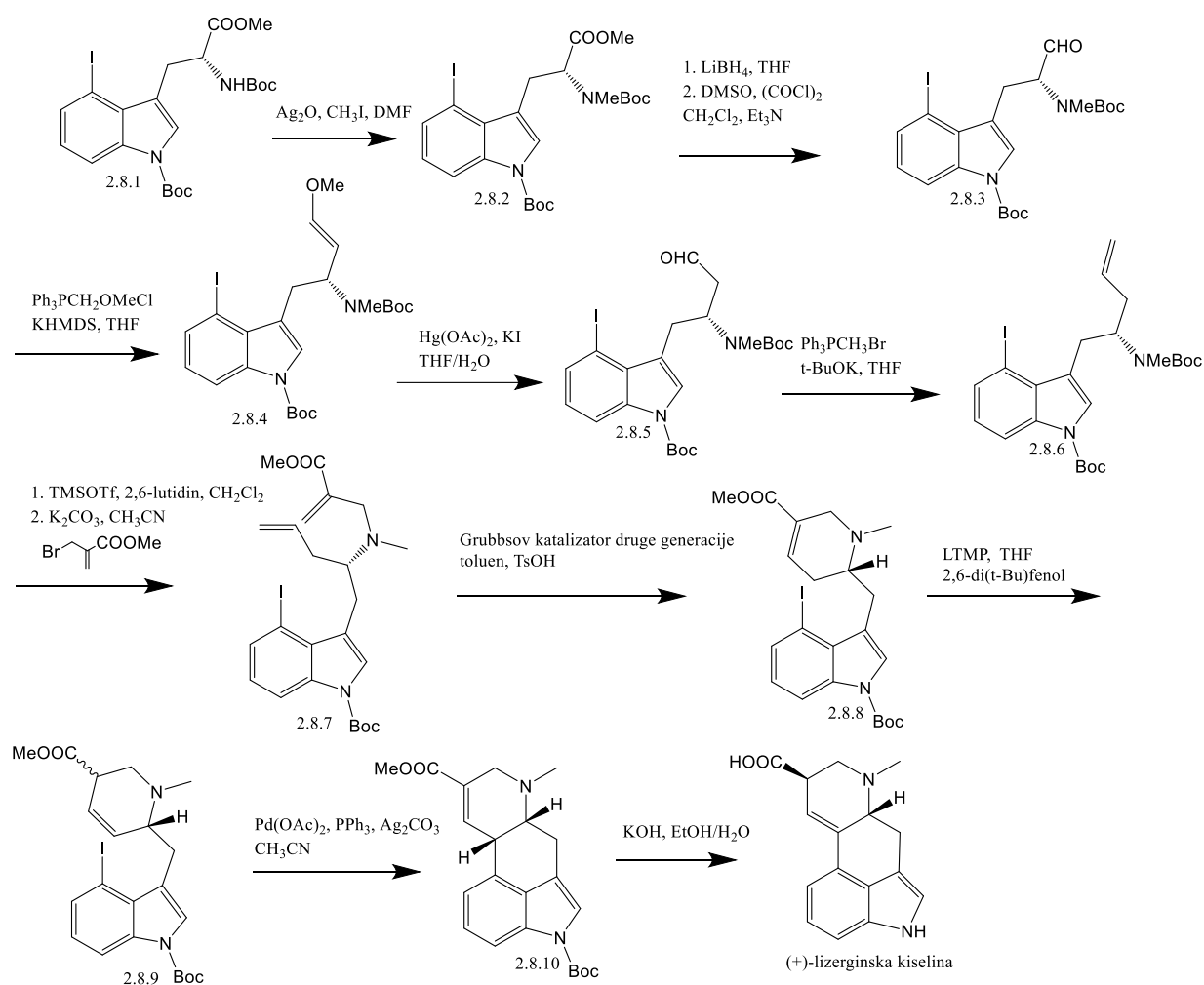
Shema 18. Sinteza lizerginske kiseline putem olefinske metateze i Heckove reakcije prema
