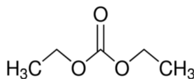
b) dietilkarbonat(DEC)
