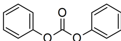
c) difenilkarbonat(DPC)
