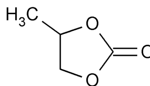
b) Propilen karbonat (PC)
