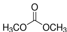
a) dimetilkarbonat(DMC)
