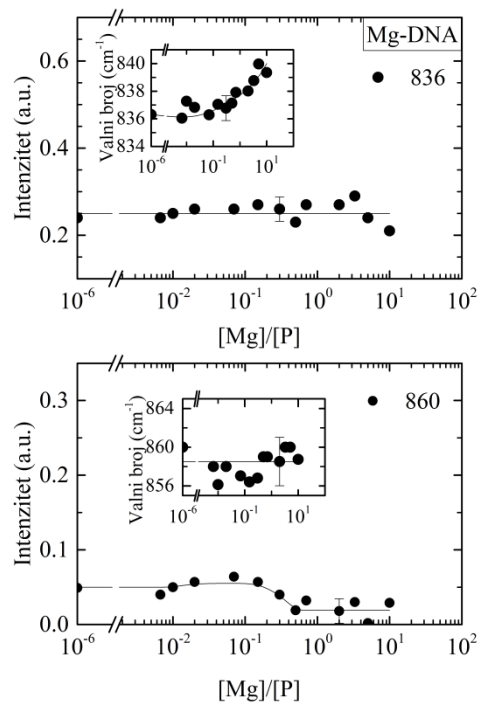
Slika 3.19 Gornja slika: Intenzitet i valni broj (umetak) B markera (836) tankih filmova Mg-DNA u MgCl 2 , kao funkcija r=[\text{Mg}]/[\text{P}] . Donja slika: Intenzitet i valni broj (umetak) A markera (860) tankih filmova Mg-DNA u MgCl 2 , kao funkcija r=[\text{Mg}]/[\text{P}] . Točke na r=10^{-6} odgovaraju referentnom uzorku Mg-DNA. Pune linije su povučene „naoko“.
