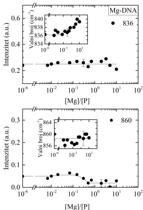
Slika 3.19 Gornja slika: Intenzitet i valni broj (umetak) B markera (836) tankih filmova Mg-DNA u \text{MgCl}_2 , kao funkcija r=[Mg]/[P] . Donja slika: Intenzitet i valni broj (umetak) A markera (860) tankih filmova Mg-DNA u \text{MgCl}_2 , kao funkcija r=[Mg]/[P] . Točke na r=10^{-6} odgovaraju referentnom uzorku Mg-DNA. Pune linije su povučene „naoko“.
