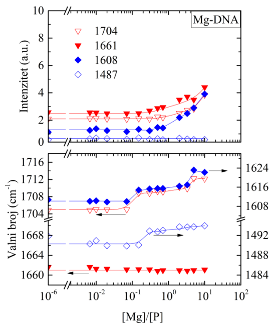
Slika 3.20 Intenzitet (gornja slika) i valni broj (donja slika) najznačajnijih vrpca baza Mg-DNA u MgCl_2 kao funkcija r=[Mg]/[P] . C=O vrpca na 1704\text{ cm}^{-1} (otvoreni crveni trokutići) i 1661\text{ cm}^{-1} (puni crveni trokutići); C=N vrpca na 1608\text{ cm}^{-1} (puni plavi rombovi) i 1487\text{ cm}^{-1} (prazni plavi rombovi). Točke na r=10^{-6} odgovaraju referentnom uzorku Mg-DNA. Pune linije su povučene „naoko“.
