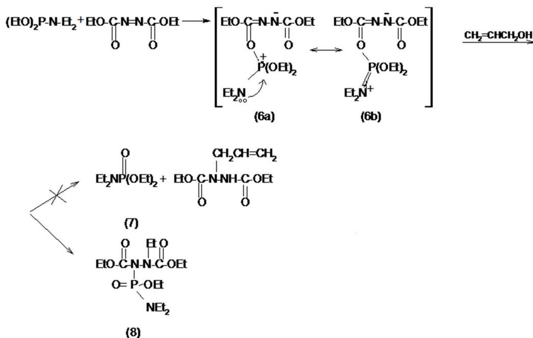
Slika 17: oksidacija trialkilfosfita
