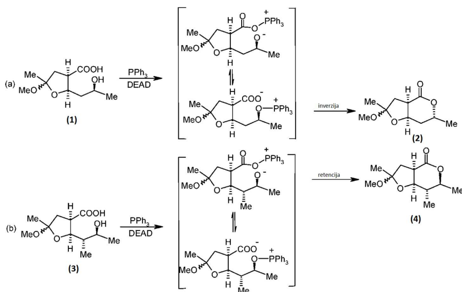
Slika 13: laktonizacija sterički zakrčenog alkohola uz retenciju konfiguracije 1
