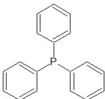
Slika 5: trifenilfosfin, PPh_3
