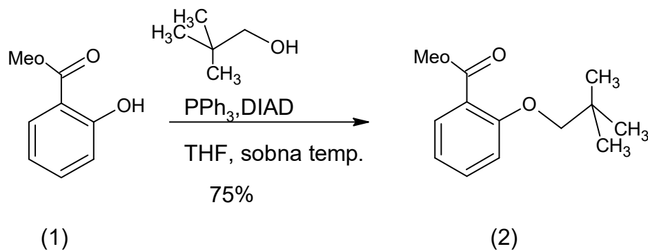
Slika 32: ultrazvukom pomognuta Mitsunobu eterifikacija pri sobnoj temperaturi
