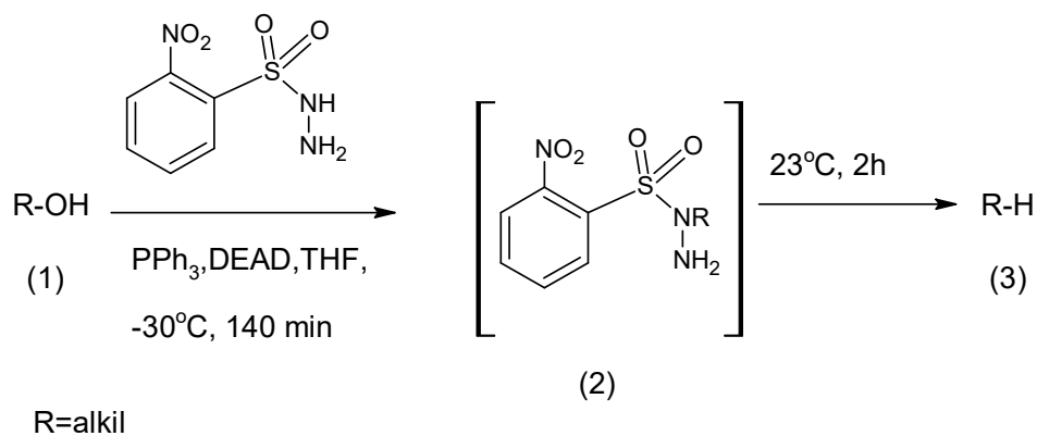
Slika 33: deoksigenacija alkohola do alkana potaknuta o -nitrobenzensulfonilhidrazinom
