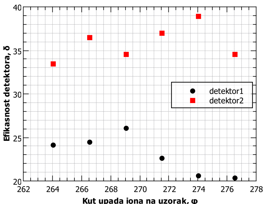
Slika 6.2: Kliracijska krivulja kuta za centriranje detektorskog sistema za maksimalnu efikasnost
