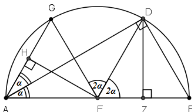
Slika 3.1: Ilustracija uz al-Kāšijev fundamentalni teorem
