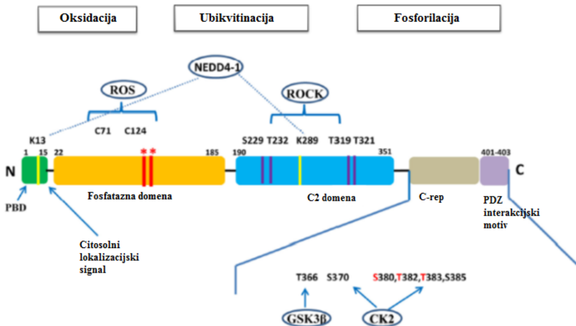
Slika 6. Shematski prikaz domena PTEN proteina: N-terminalna PIP 2 -vezujuća domena (PBD), fosfatna domena, C2 domena, C-terminalni rep fosforiliran od glikogen sintaze kinaze 3 \beta (GSK3 \beta ) i PDZ-međureakcijski motiv. Mutacije koje onemogućuju fosfatnu aktivnost prikazane na slici su C124S (lipid- i protein- fosfatna aktivnost) i G129E (lipid-fosfatna aktivnost). Mutacije na položajima S380, T382 i T383 mogu destabilizirati PTEN i pojačati fosfatnu aktivnost. Na položajima K13 i K2289 dolazi do ubikvitinacije PTEN-a 27 .
