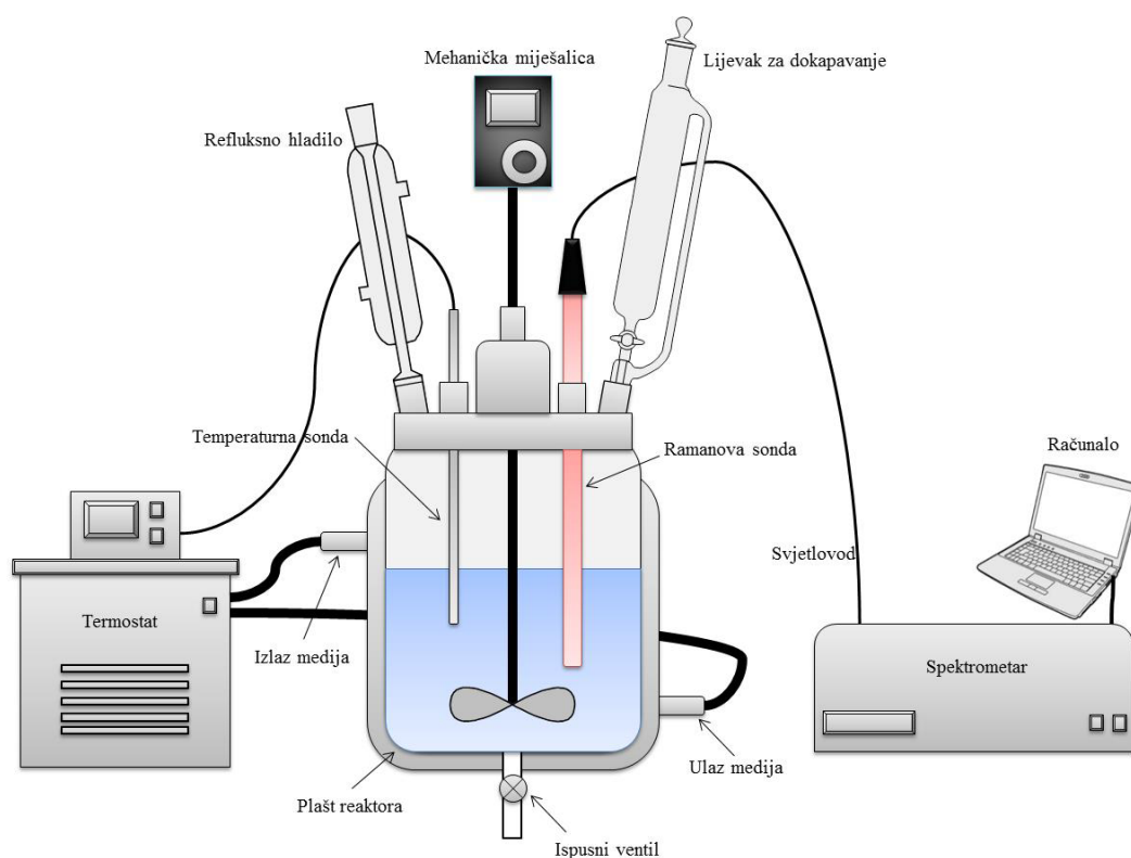
Slika 3.1. Shematski prikaz aparature korištene tijekom priprave spoja 2 i praćenja reakcije oksidacije in-line .
