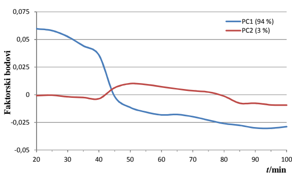
Slika 4.53. Faktorski bodovi PC1 i PC2 kroz vrijeme dobivenih PCA analizom obrađenih Ramanovih spektara in-line tijekom kalibracijskog eksperimenta 6.
