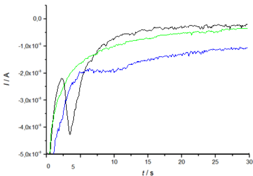
Slika 26. Kronoamperogrami snimljeni u prisutnosti Cd 2+ i HS - koncentracije 5×10 -5 mol dm -3 u 0,11 mol dm -3 NaCl pri E = -1,6 V (crna krivulja), E = -1,7 V (plava krivulja) i E = -1,8 V (zelena krivulja) t = 30 s uz t_s = 0,1 s
