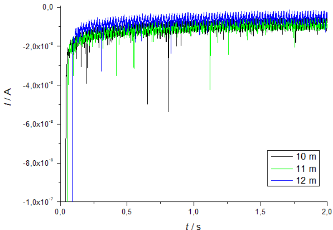
Slika 55. Kronoamperogrami snimljeni u uzorcim vodenog stupca RJ 03/2016. koji su zakisljeni do \text{pH} = 2 na E = -0,8 \text{ V} t = 2 \text{ s} uz t_s = 0,0004 \text{ s} .
