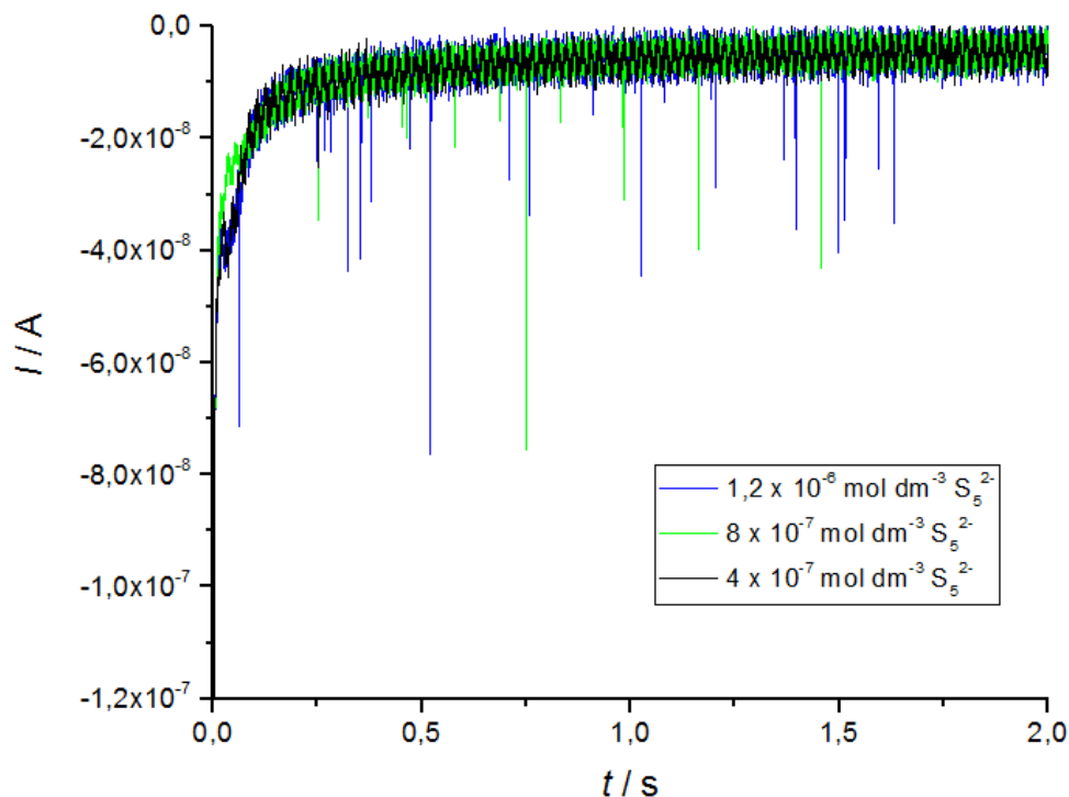
Slika 37. Kronoamperogrami snimljeni u zakiseljenoj otopini (pH = 2) S 5 2- koncentracije 4x10 -7 mol dm -3 (crna krivulja), 8x10 -7 mol dm -3 (zeleno krivulja) i 1,2x10 -6 mol dm -3 (plava krivulja), t = 2 s uz t s = 0,0004 s
